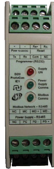
Optional protocol converter
